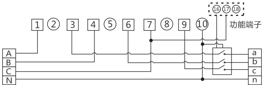
三相四线直接式接线图
