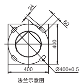
法兰示意图
