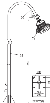
法兰式(f)
