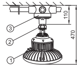
吸顶式(x)
