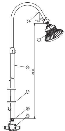
弯杆式(w)
