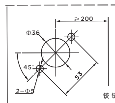
圆形延伸旋转手柄开孔尺寸图
