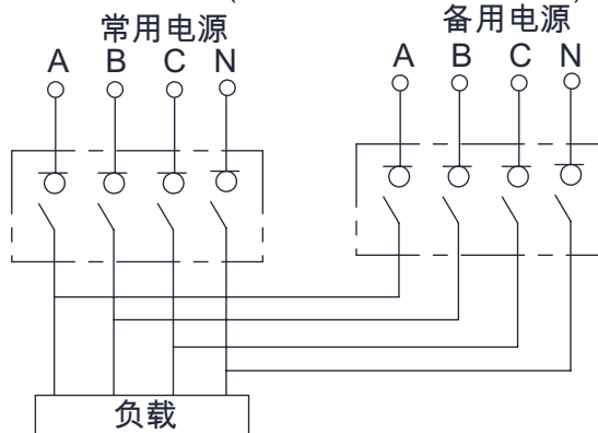
4极主回路接线（常、备电源相序必须一致）
