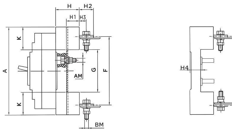
RDM5L系列插入式板后外形尺寸及安装板开孔尺寸图
