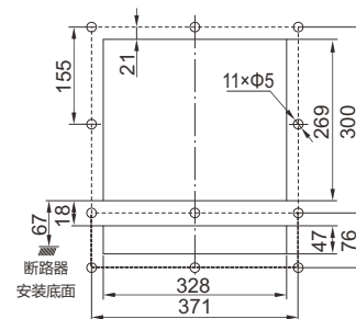
RDW7-6300抽屉式门框开孔尺寸
