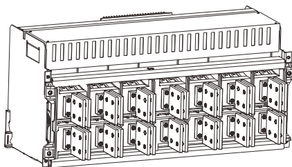
RDW7-6300/4P 抽屉式垂直接线
