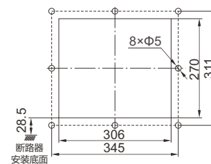
RDW7-2500固定式门框开孔尺寸
