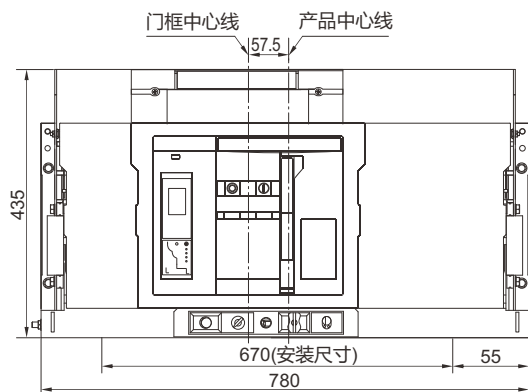
RDW7-6300/3P 抽屉式水平接线
