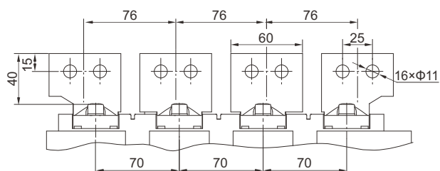
垂直接线及相间距
