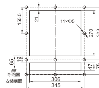
RDW7-2500S抽屉式门框开孔尺寸
