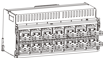
RDW7-6300/4P 抽屉式水平接线
