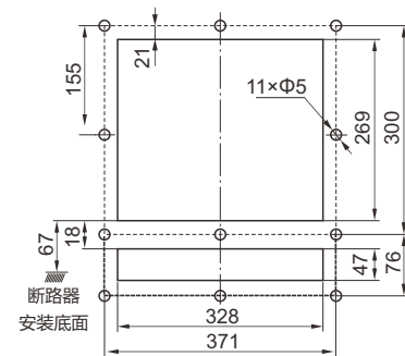
RDW7-4000S抽屉式门框开孔尺寸
