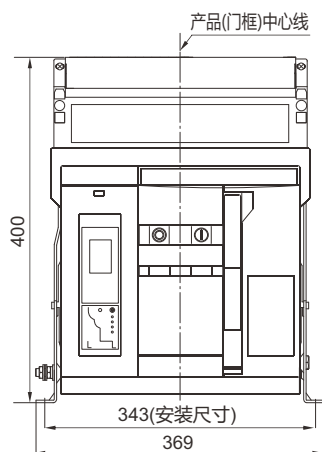
外形尺寸
