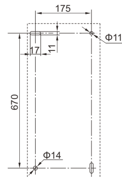
RDW7-6300抽屉式门框开孔尺寸
