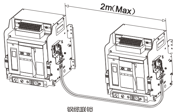
钢缆联锁
