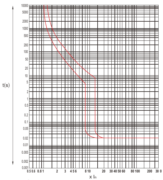
RDM7L-250 时间/电流特性曲线
