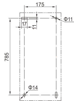
RDW7-6300抽屉式门框开孔尺寸
