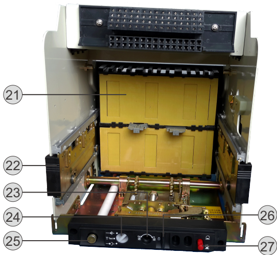
抽屉座
