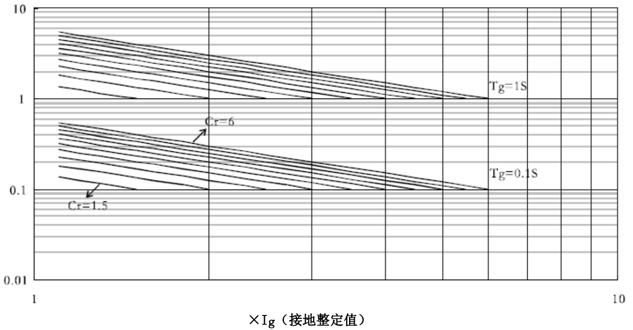
接地保护
