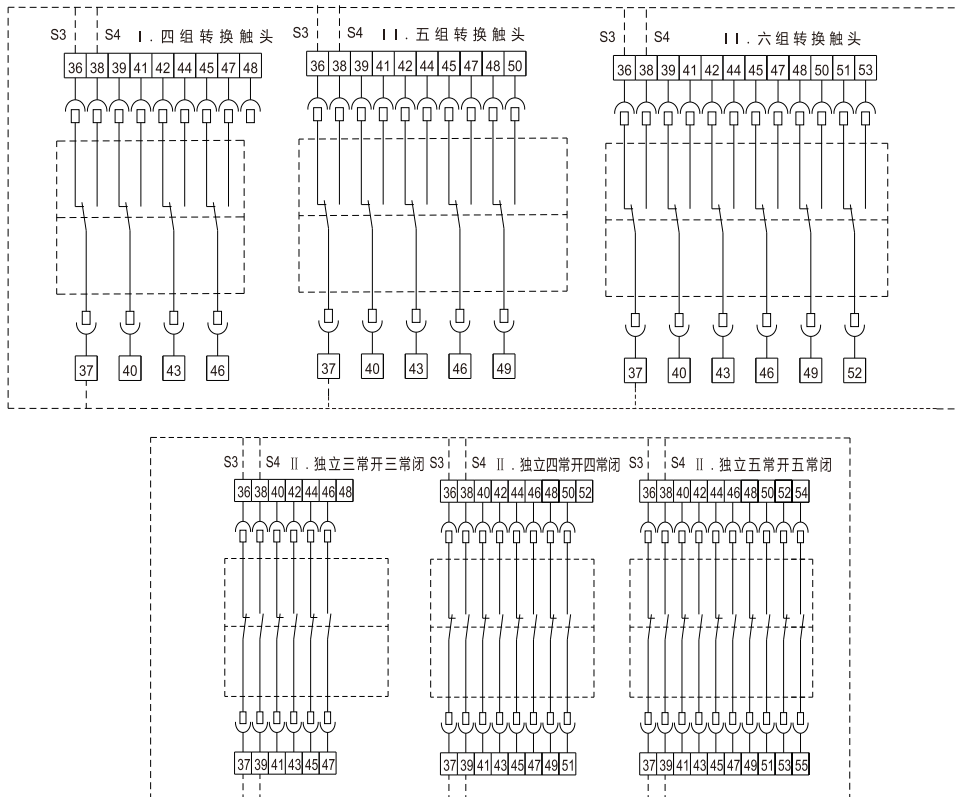
RDW8HU-2500/4000/6300 M型二次回路接线图端子功能与符号释义
