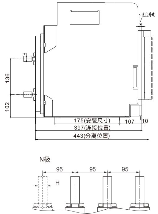
垂直接线及相间距（长排）
