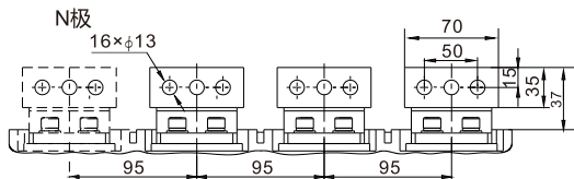
水平接线及相间距（短排）
