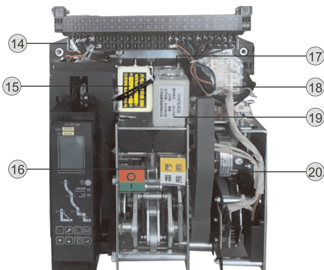
断路器本体
