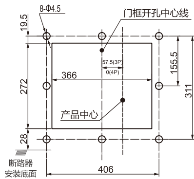
RDW8HU-6300固定式断路器面板开孔尺寸
