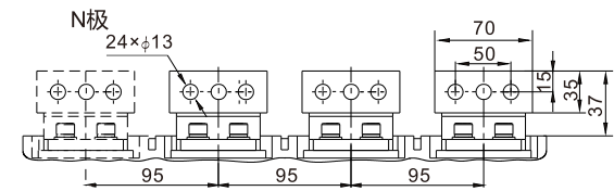
水平接线及相间距（短排）
