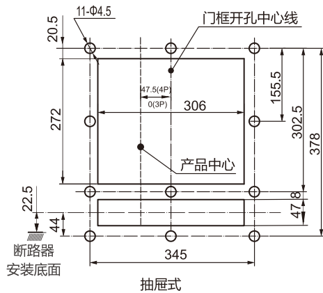
RDW8HU-2500抽屉式断路器面板开孔尺寸
