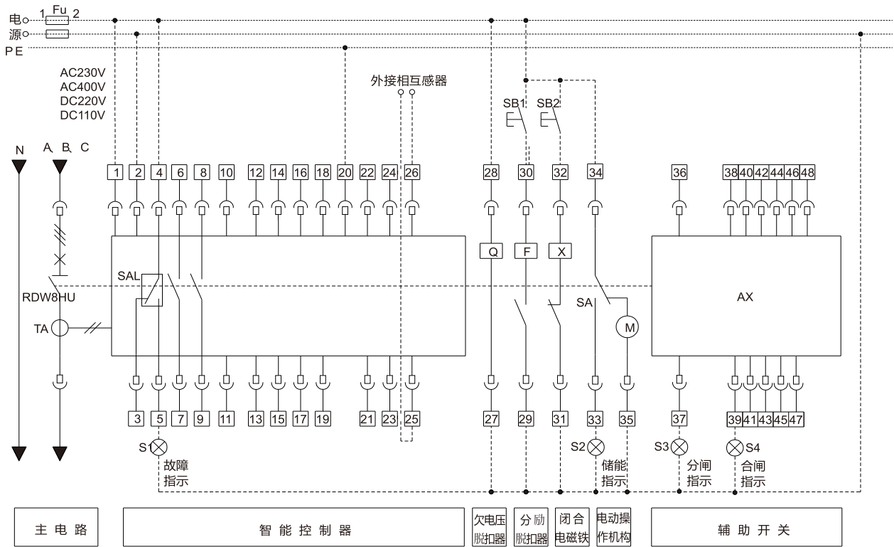
RDW8HU-2500/4000/6300 R型二次回路接线图
