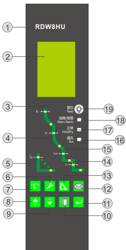
RDW8HU智能控制器界面
