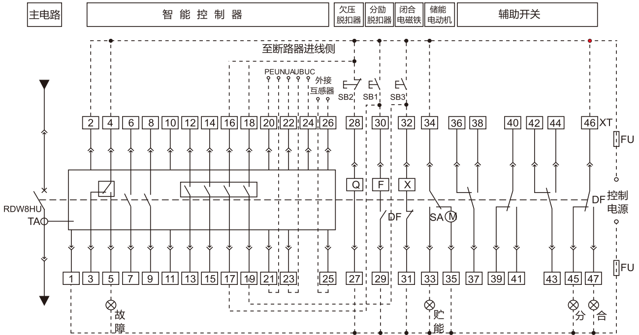
RDW8HU-2500-6300带重合闸功能断路器控制回路接线图
