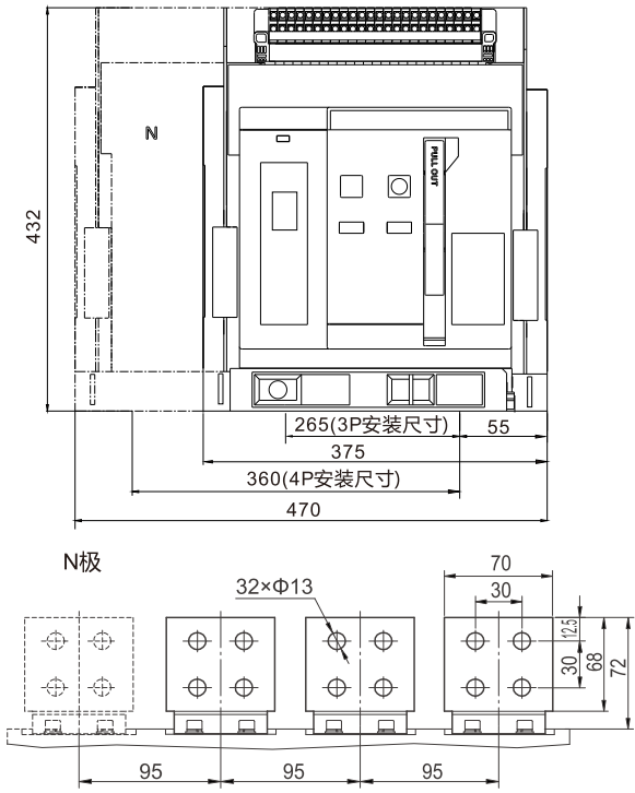
默认出厂：水平接线及相间距（长排）
