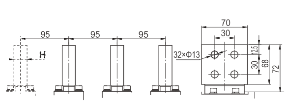
垂直接线及相间距
