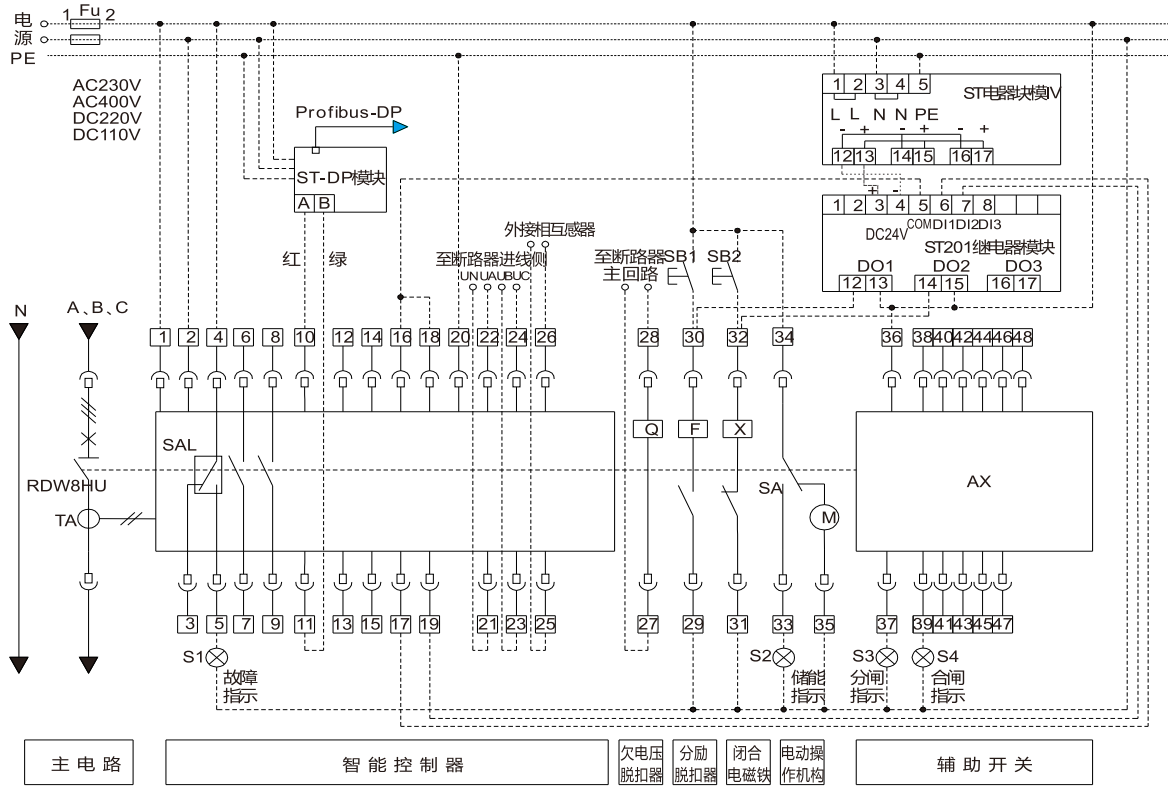
RDW8HU-2500/4000/6300 H型二次回路接线图
