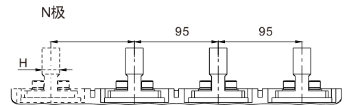
垂直接线及相间距（长排）
