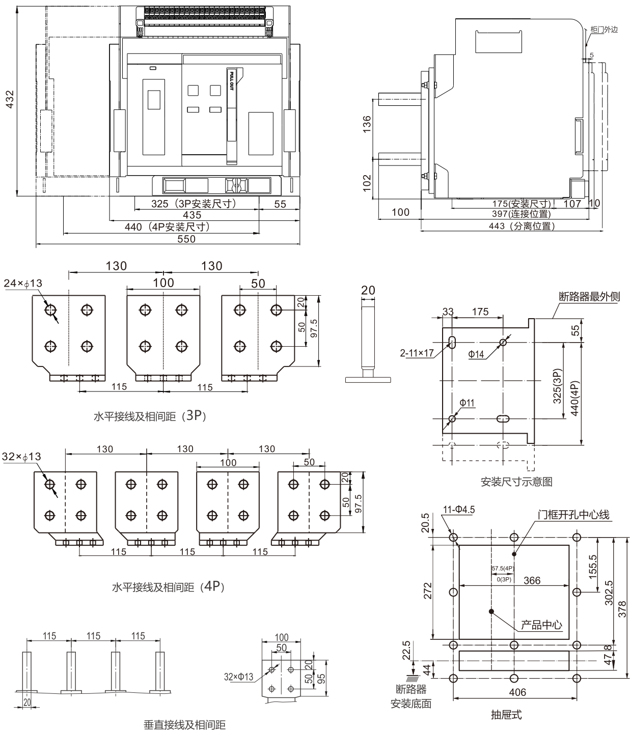
RDW8HU-4000抽屉式断路器面板开孔尺寸
