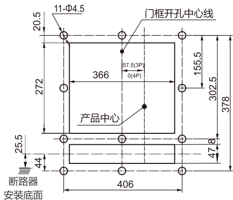
RDW8HU-6300抽屉式断路器面板开孔尺寸
