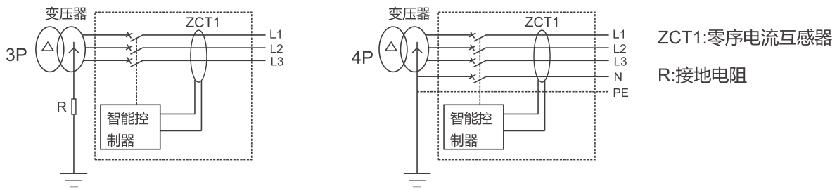
剩余电流保护电气原理图
