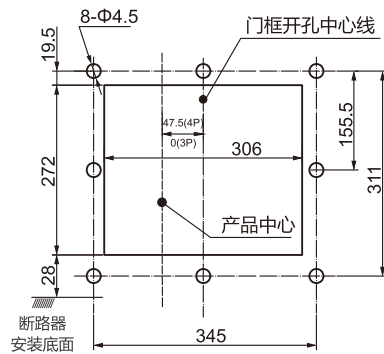
RDW8HU-2500固定式断路器面板开孔尺寸
