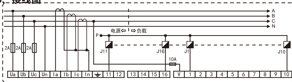
JKWRF型接线图
