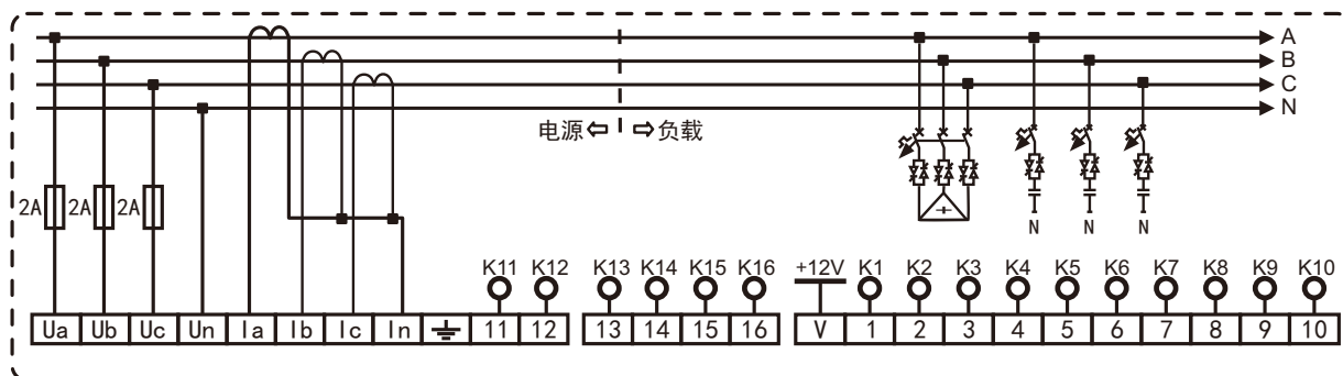
JKWRF型接线图 动态输出
