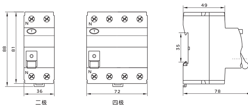
图2 RDX16L外形尺寸及安装尺寸
